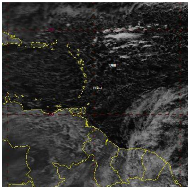
Satellitenbild Meteosat 13.01.2020 18 UTC
