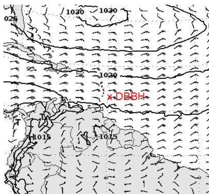
Vorhersage für Dienstag 12 UTC
