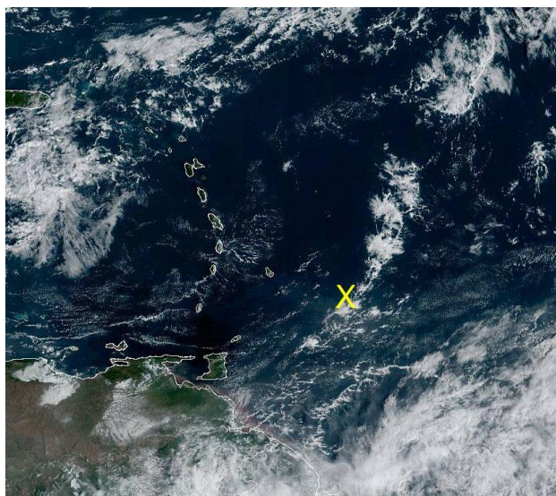
Satellitenbild GOES 27.01.2020 13:00 UTC
