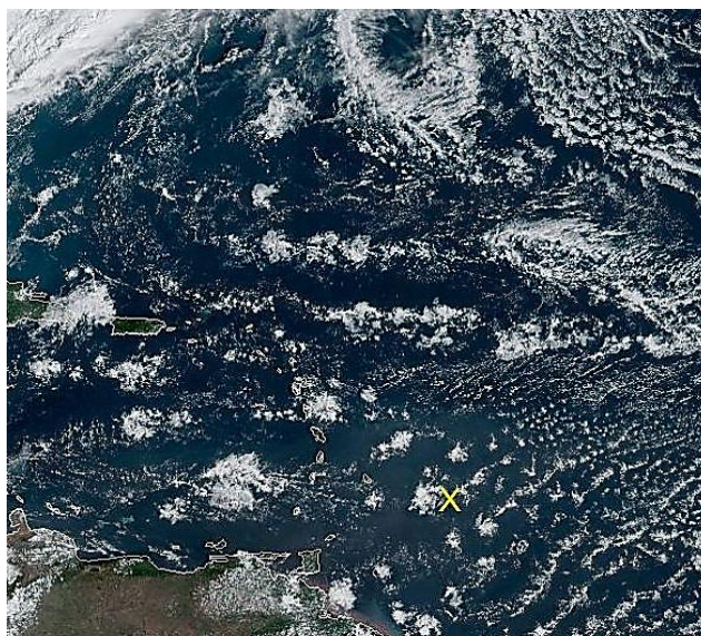
Satellitenbild GOES16 02.02.2020 13:30 UTC
