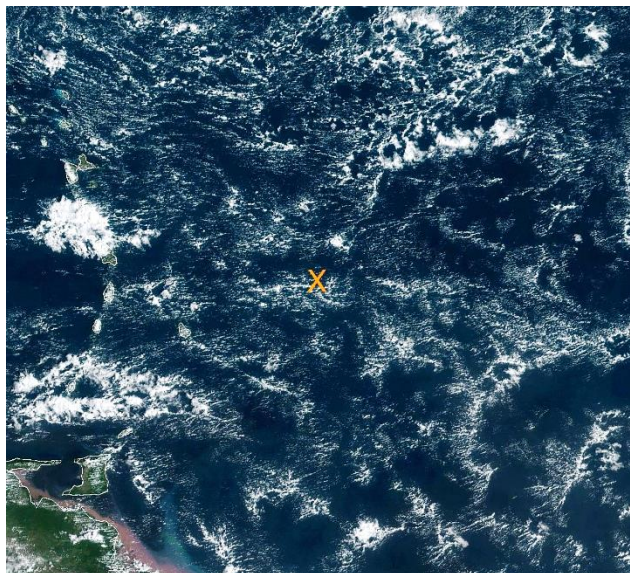
Satellitenbild GOES16 06.02.2020 12:50 UTC
