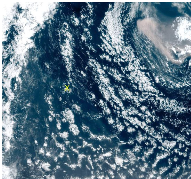
Satellitenbild GOES16 23.02.2020 13.20 UTC
