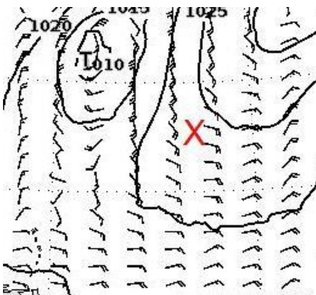
Vorhersage für Montag 12 UTC
