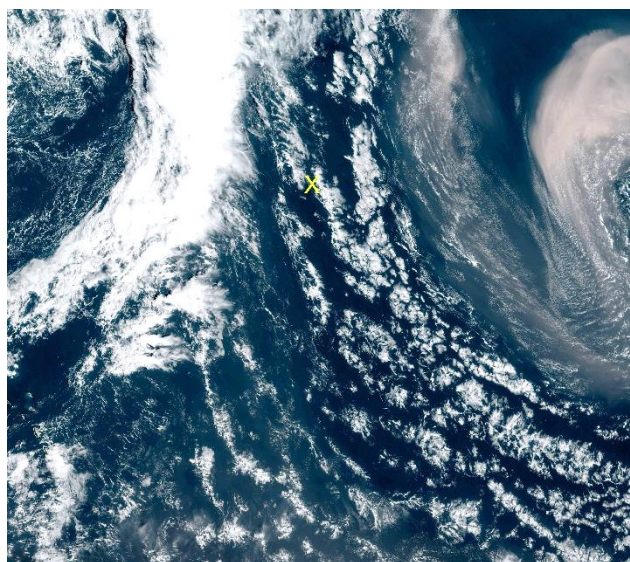
Satellitenbild GOES16 24.02.2020 13:20 UTC
